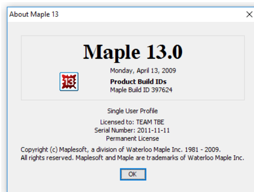
Gambar 1. Maple versi 13
