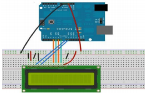
Gambar 3. Arduino dengan LCD 16 x 2
