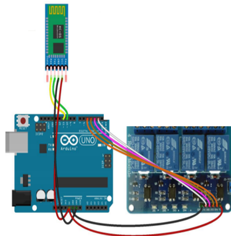
Gambar 13. Rancangan Alat Keseluruhan
