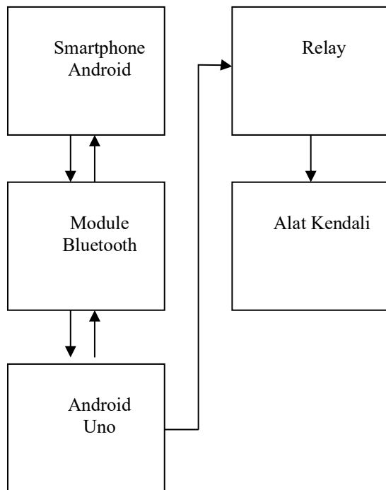
Gambar 8. Blok Diagram Dan Cara Kerja
