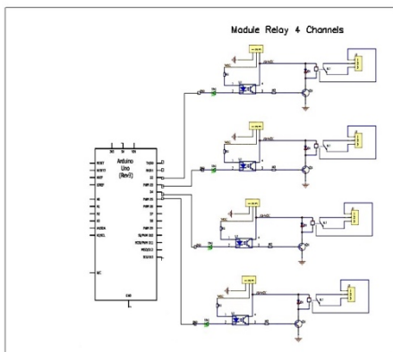
Gambar 11. Skema Rangkaian Relay dengan Arduino
