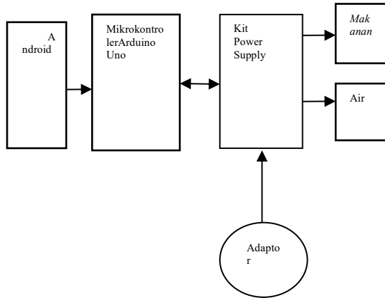
Gambar 7. Diagram Blok Rangkaian
