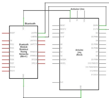
Gambar 12. Skema Rangkaian Module Bluetooth dengan Arduino
