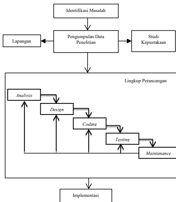
Gambar 2. Kerangka Penelitian
