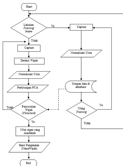
Gambar 11. Flowchart Aplikasi
