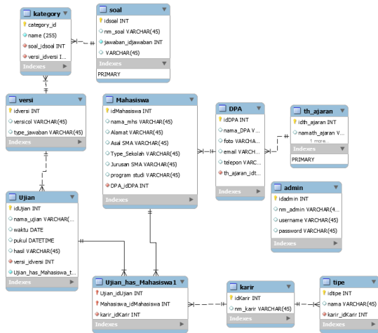
Gambar 1. Perancangan Database
