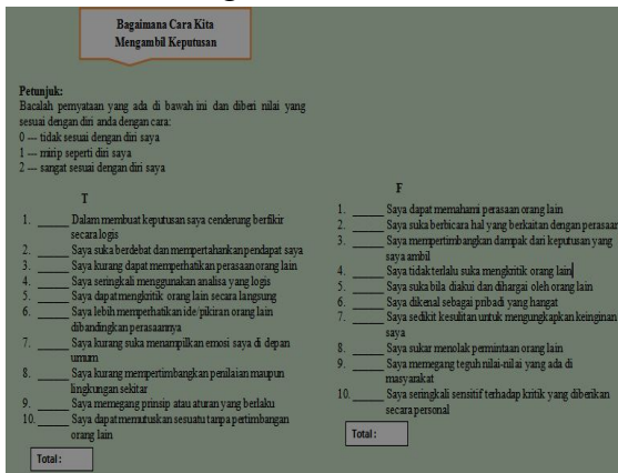
Gambar 2. Pengukuran MBTI
